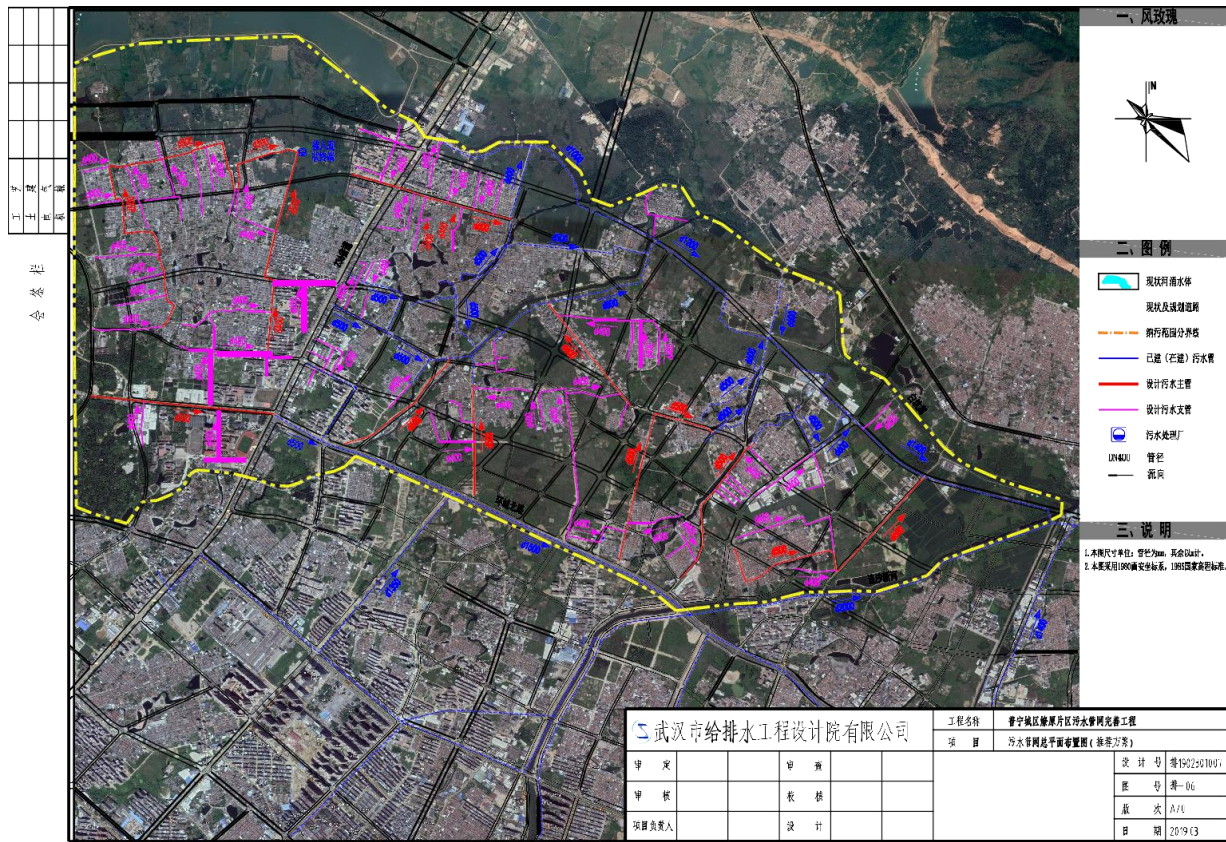
图 1-1 管网布置示意图 (蓝色：现状污水管，红色：设计污水干管)
